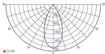
Lichtverteilungskurve
